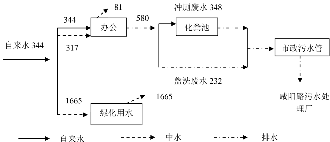
图 2-1 本项目水平衡图 (m³/a)
